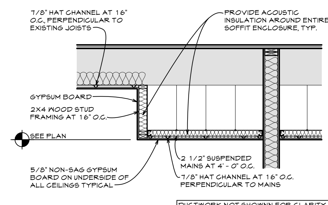
2 SOFFIT DETAIL SCALE: 1/2" = 1'-0"
