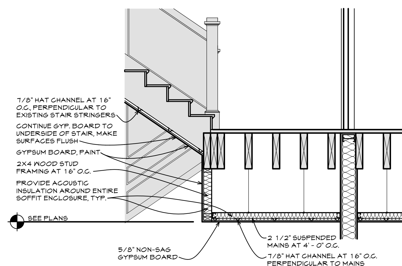
1 SOFFIT DETAIL SCALE: 1/2" = 1'-0"
