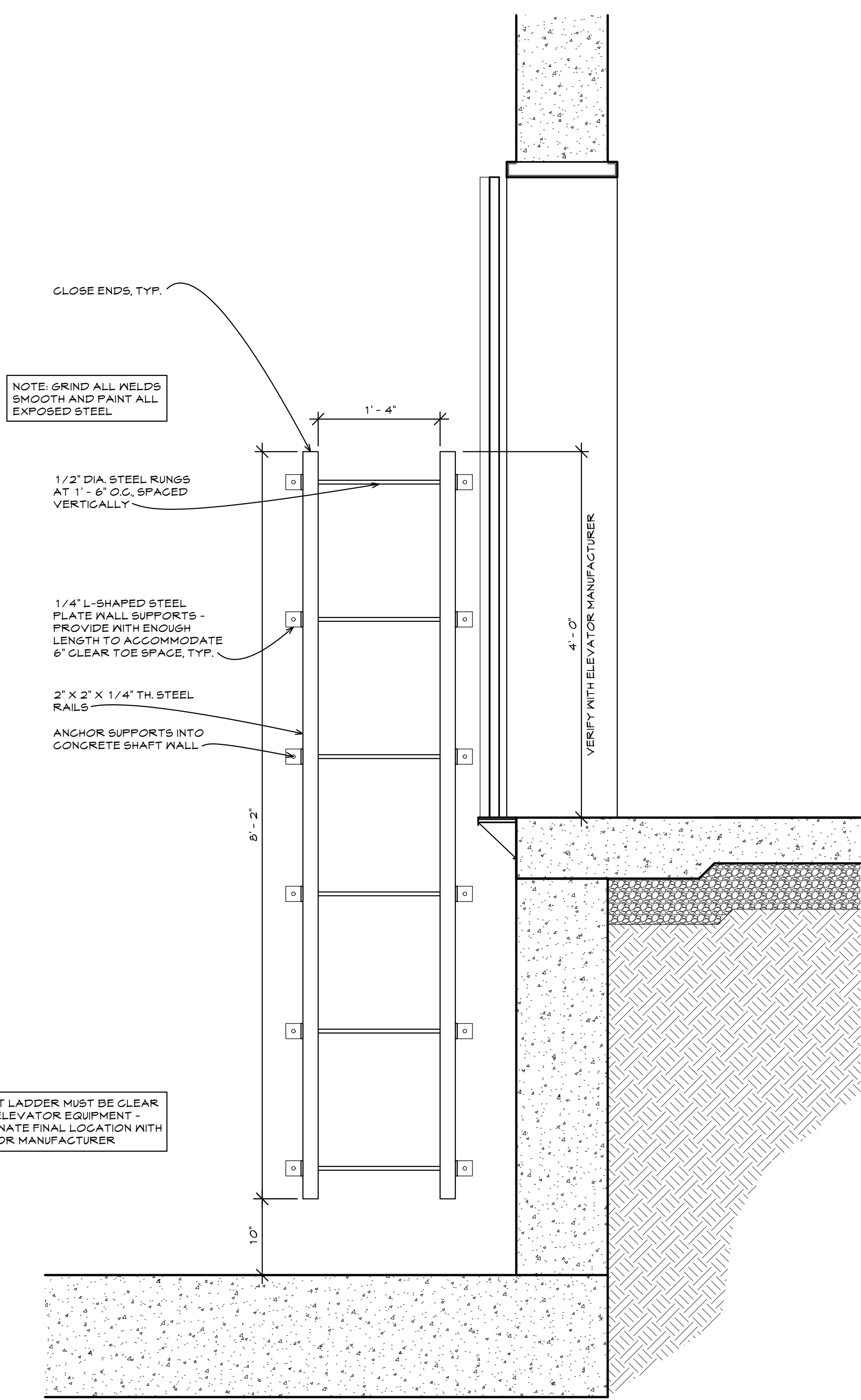
② PIT LADDER SCALE: 1" = 1'-0"
